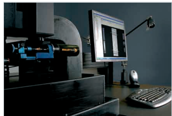
BulletTRAX-3D, estación de captura de imágenes 3D de Forensic Technology.
